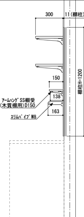
B-B' 断面
