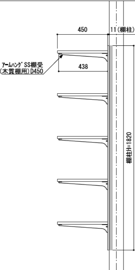
A-A' 断面
