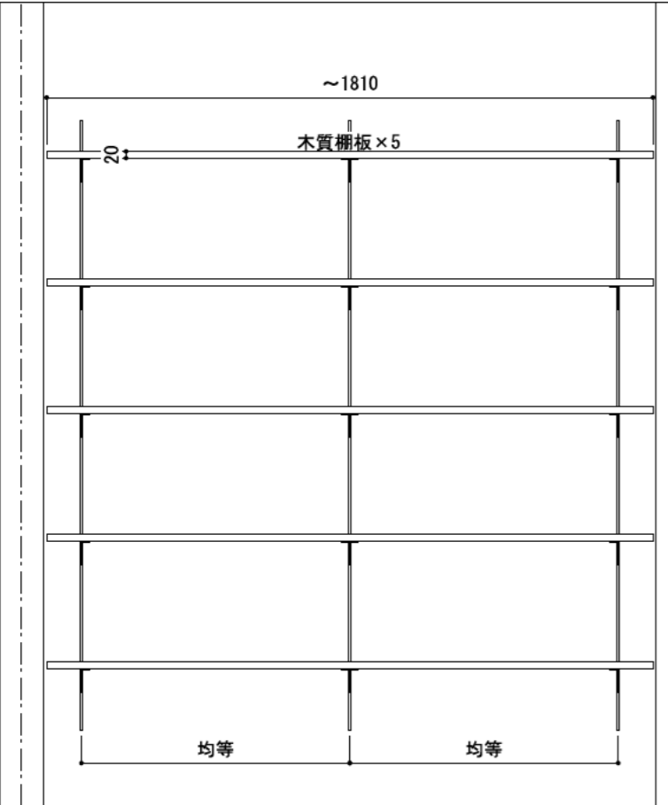
A立面
