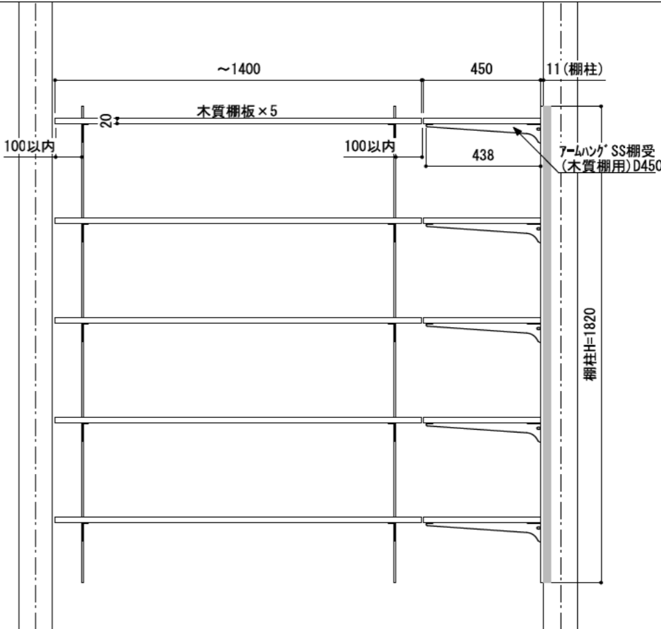
B-B' 断面
