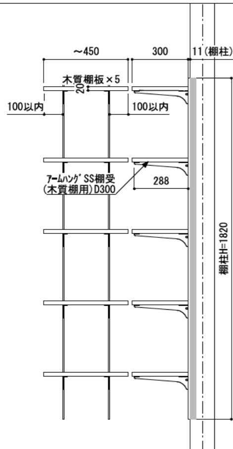
B立面
