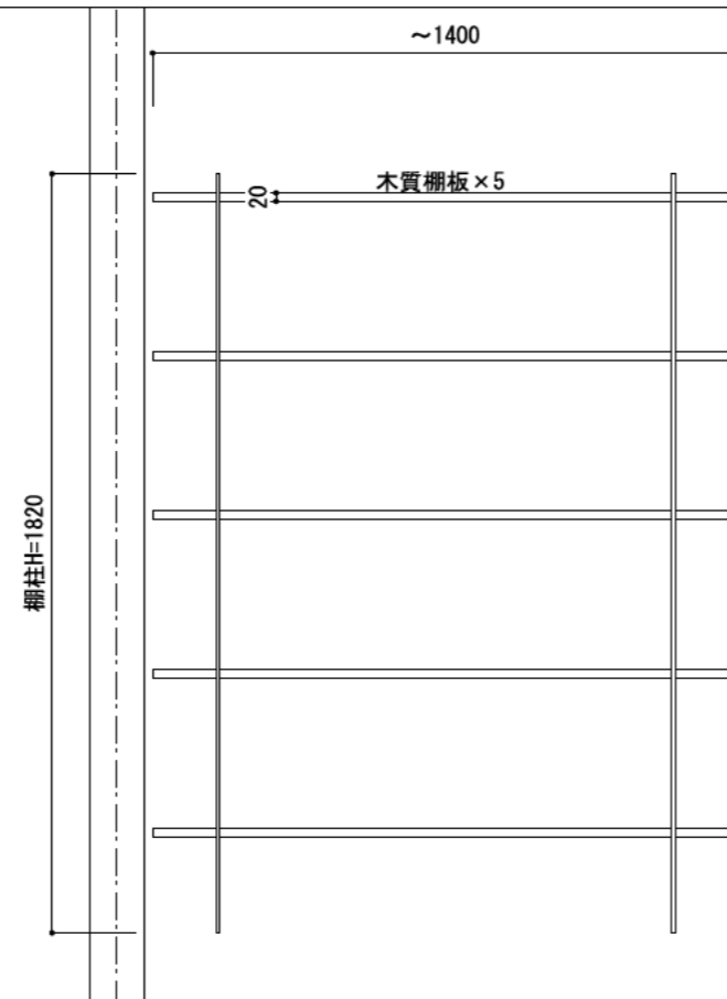
A立面
