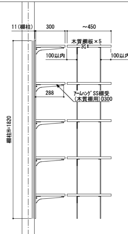
C立面
