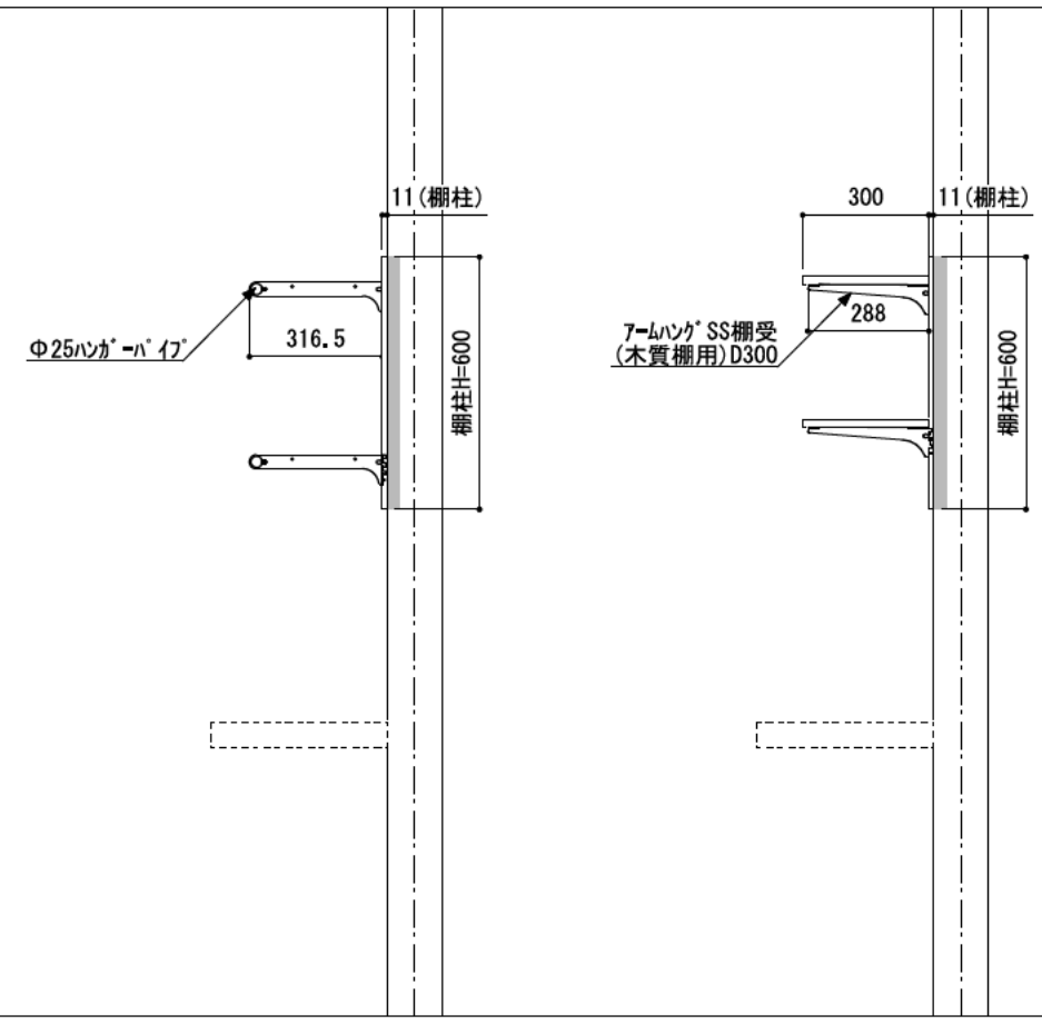
A-A' 断面
