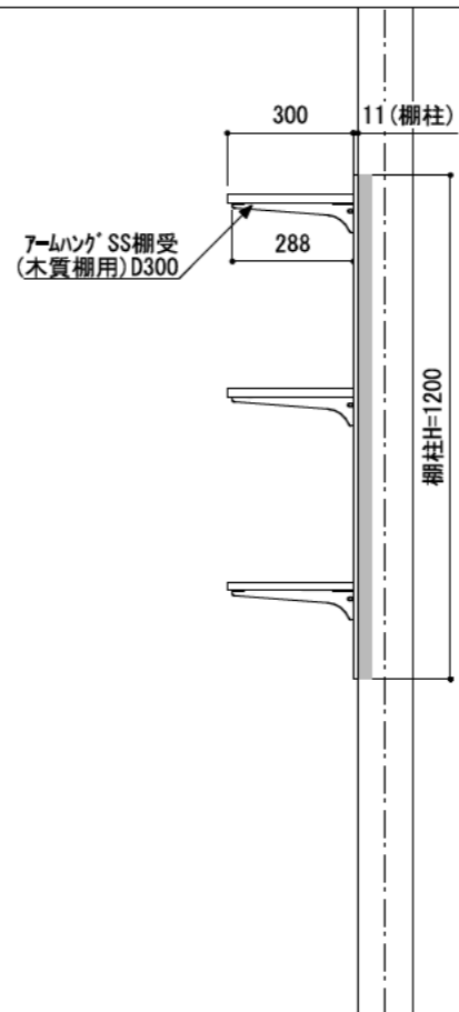
A-A' 断面
