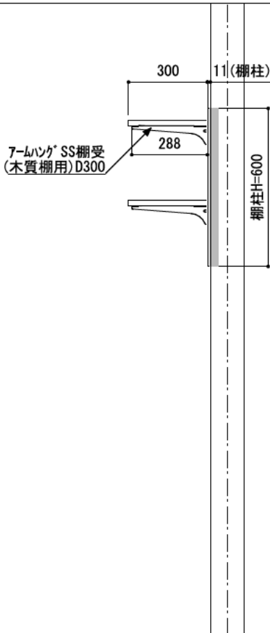
A-A' 断面
