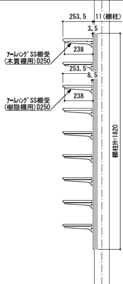
A-A' 断面
