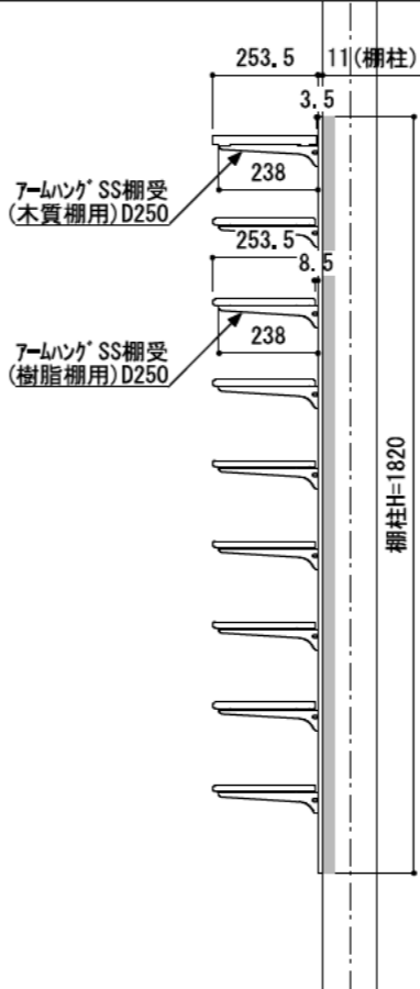
A-A' 断面
