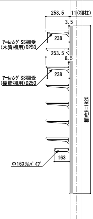
B-B' 断面
