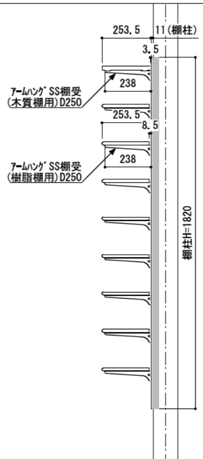
A-A' 断面
