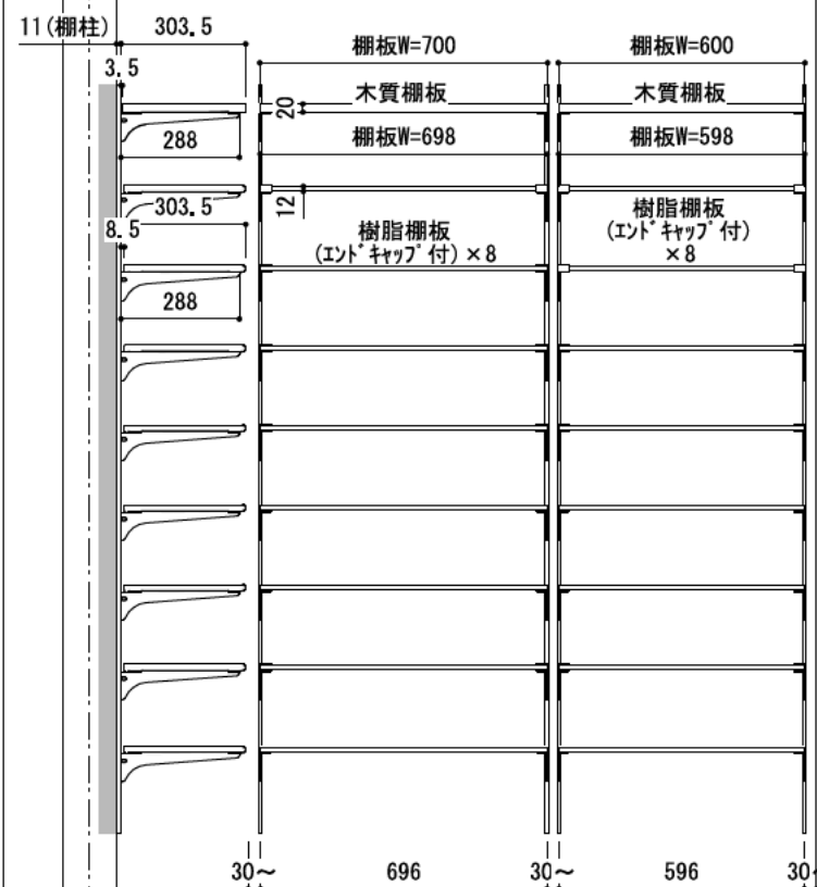
B立面 AG000073 ■ □
