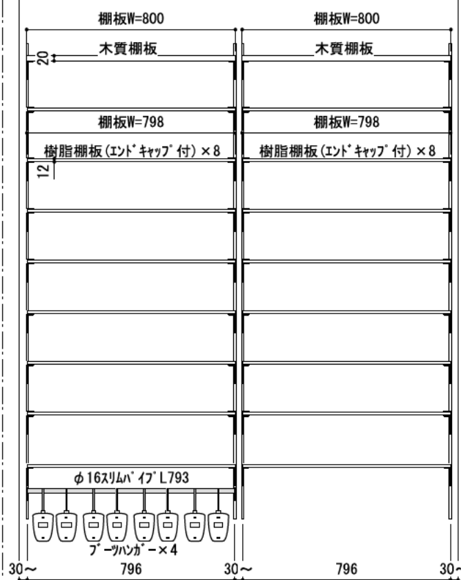
A立面 AG000067 ■ □
