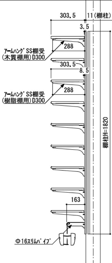
A-A' 断面
