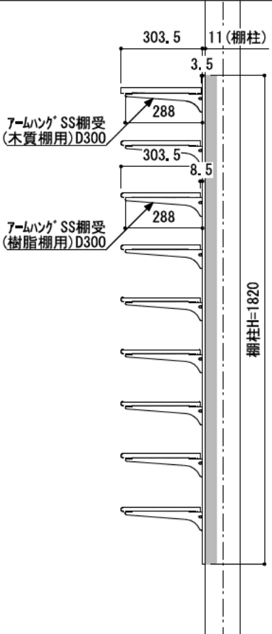
B-B' 断面
