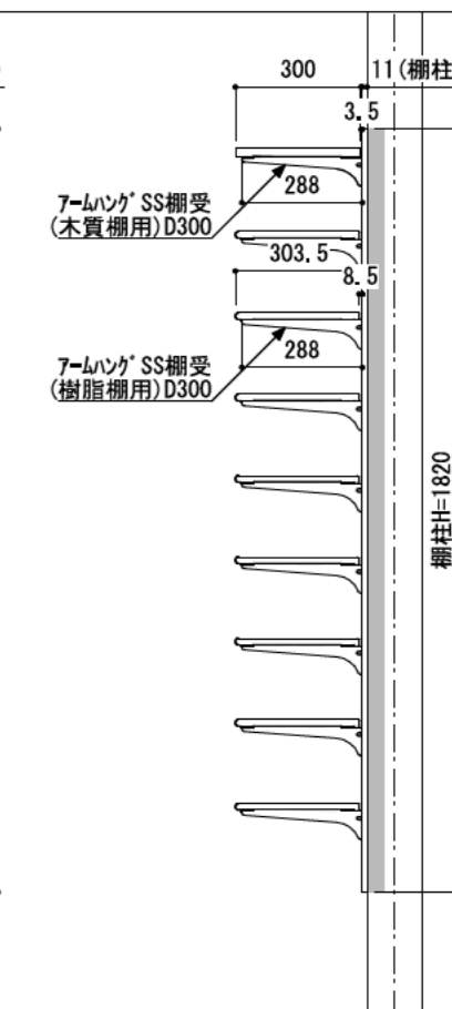
C-C' 断面
