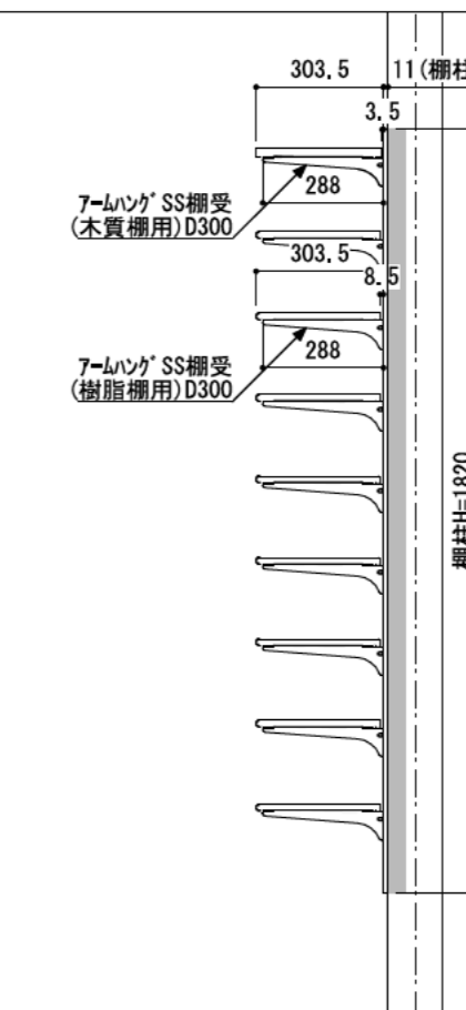
B-B' 断面
