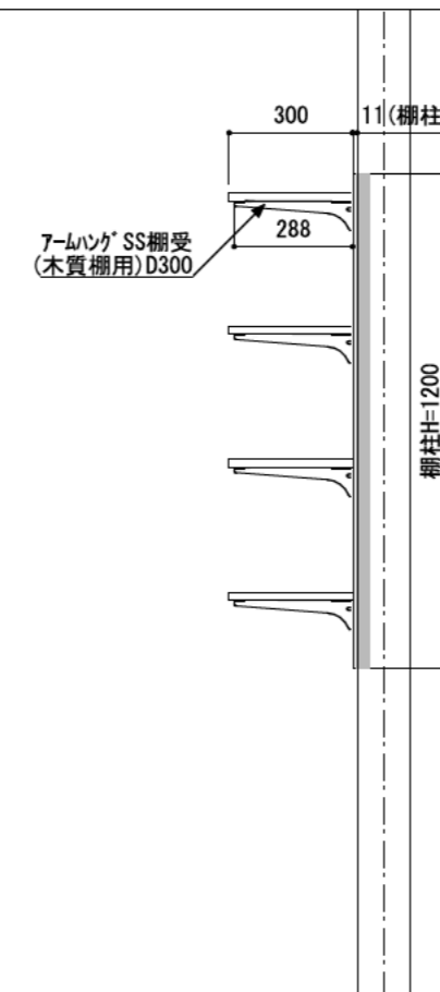
A-A' 断面
