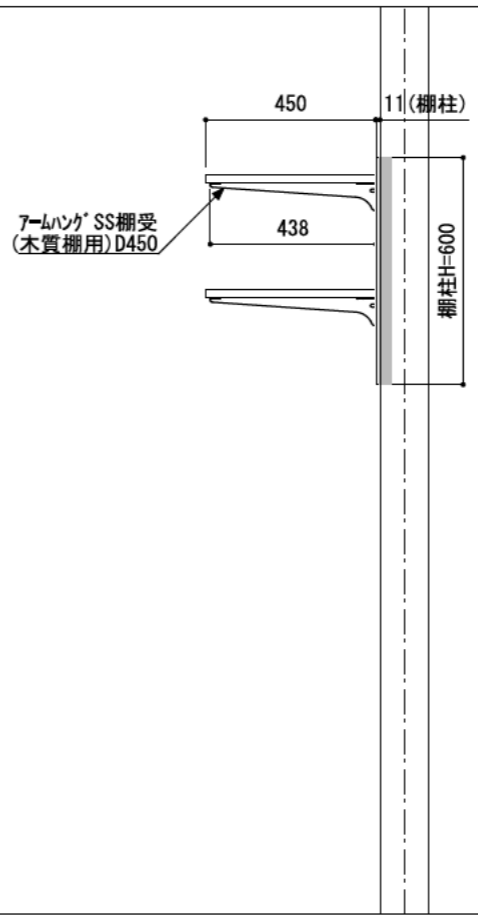
A-A' 断面
