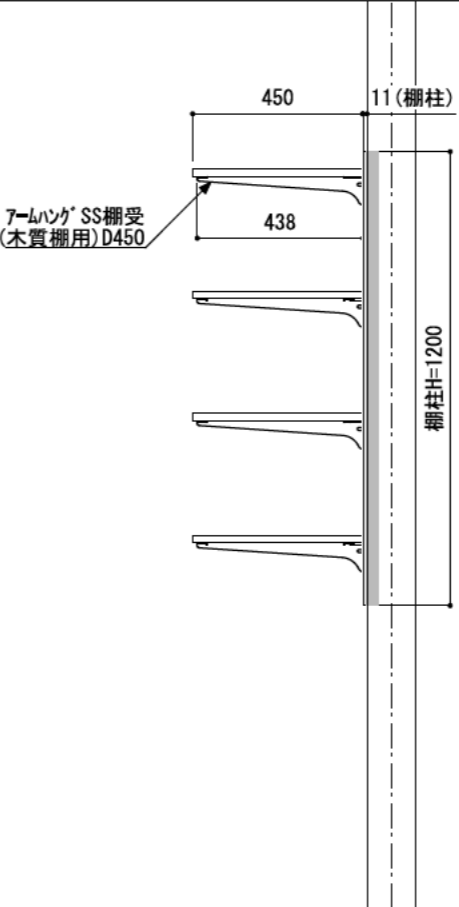
A-A' 断面
