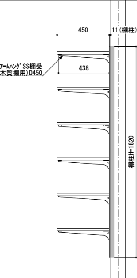
A-A' 断面
