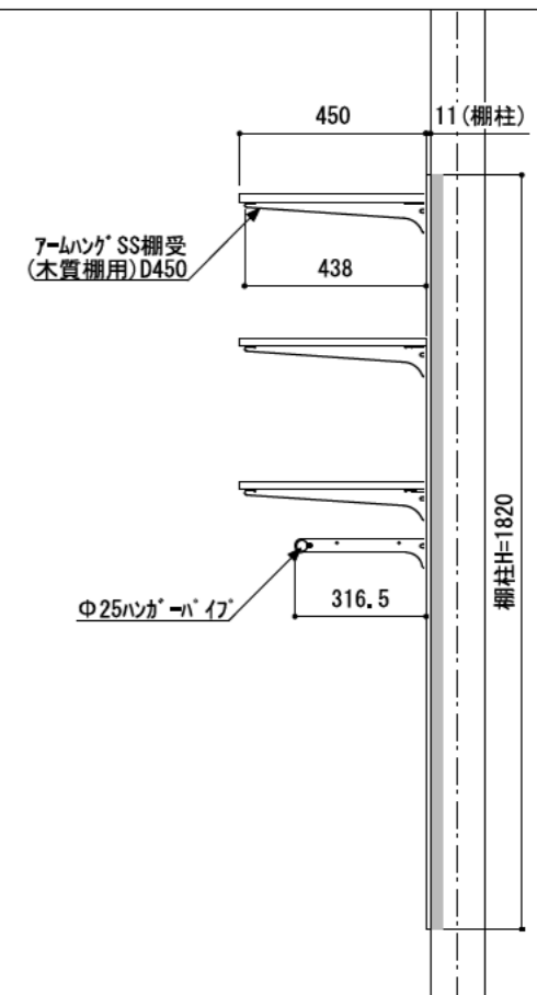
B-B' 断面
