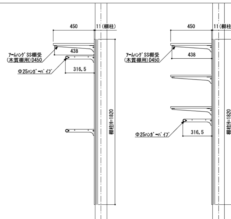
A-A' 断面
