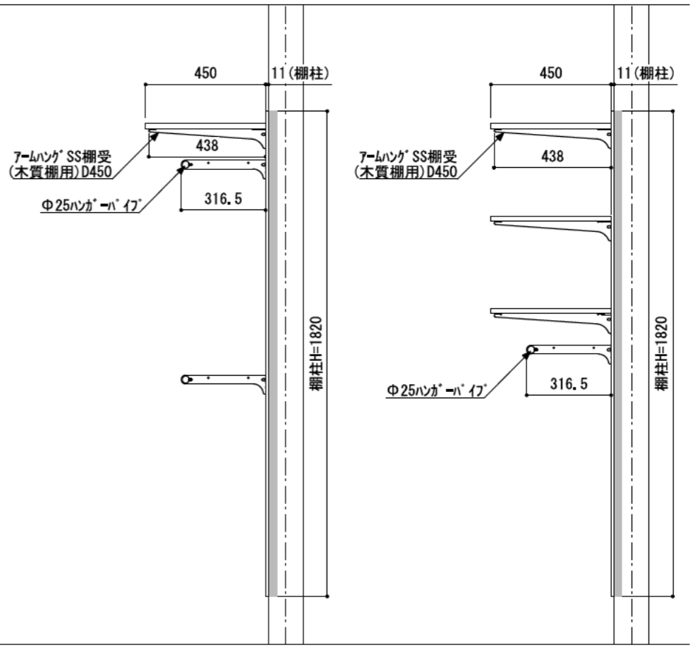
A-A' 断面
