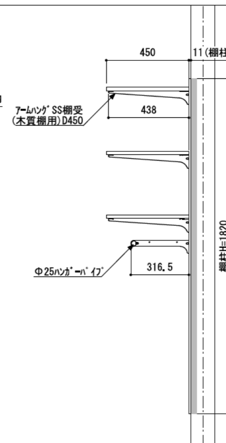
A-A' 断面
