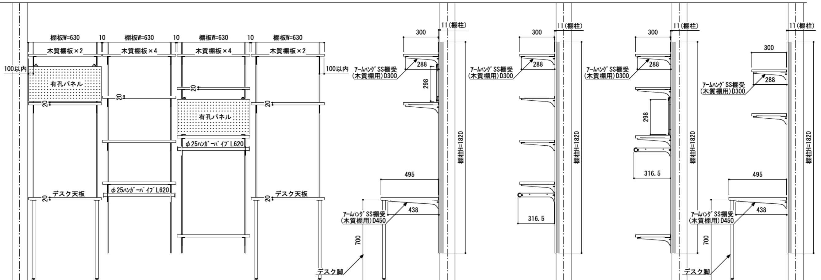
A-A' 断面
