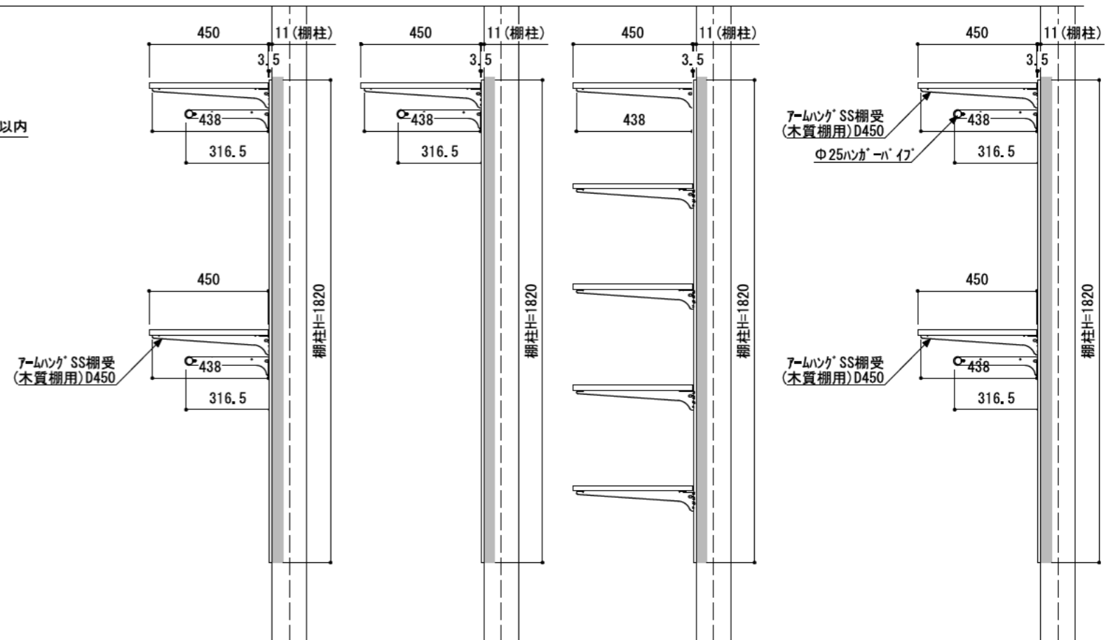
A-A' 断面
