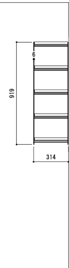
A-A' 断面
