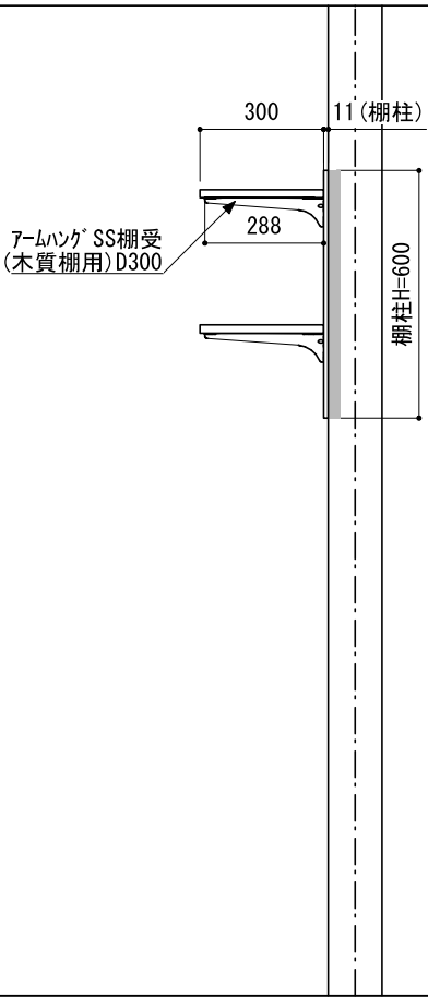
A-A' 断面
