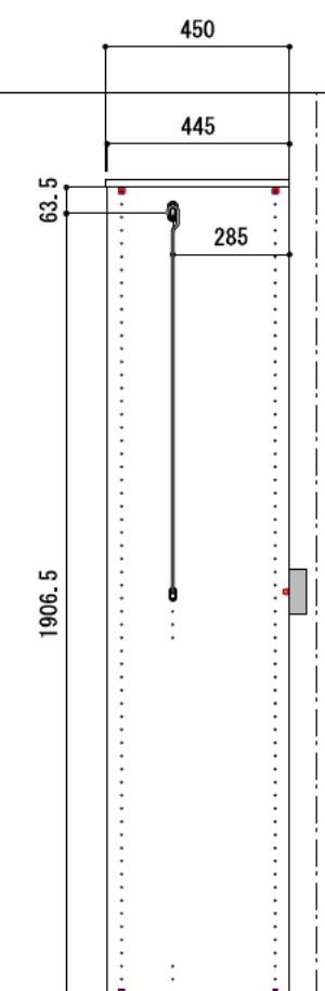
A-A' 断面
