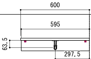
A-A' 断面
