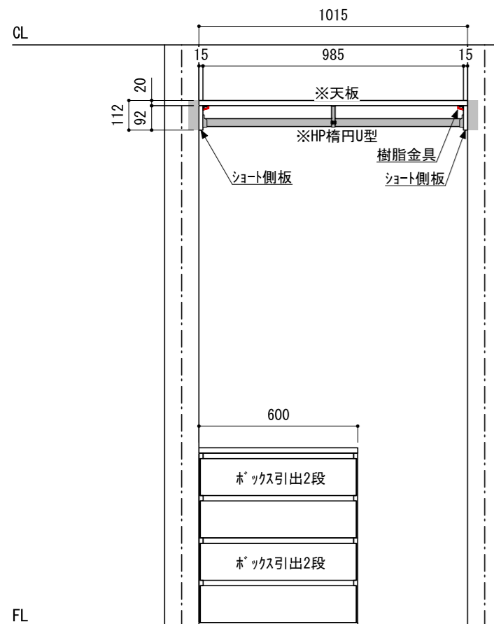
②立面
