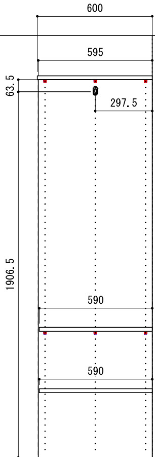
D-D' 断面
