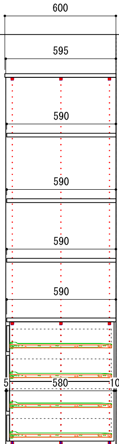
E-E' 断面
