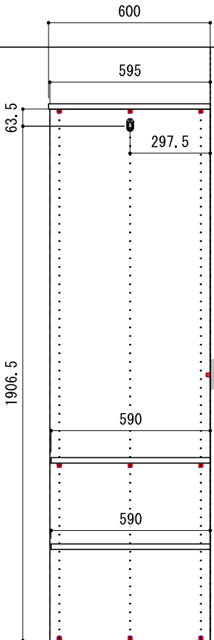
C-C' 断面
