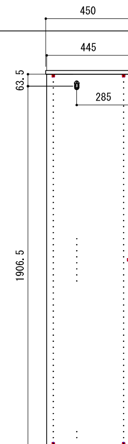
A-A' 断面
