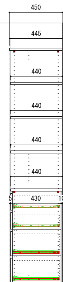
A-A' 断面
