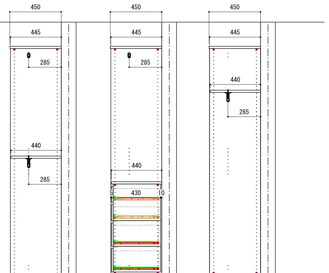
A-A' 断面
