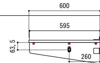
B-B' 断面
