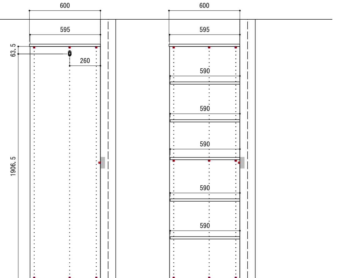
A-A' 断面
