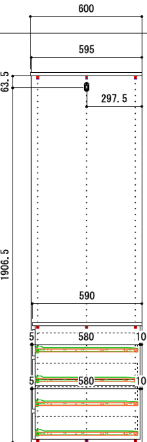
B-B' 断面
