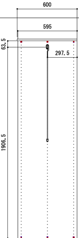
C-C' 断面
