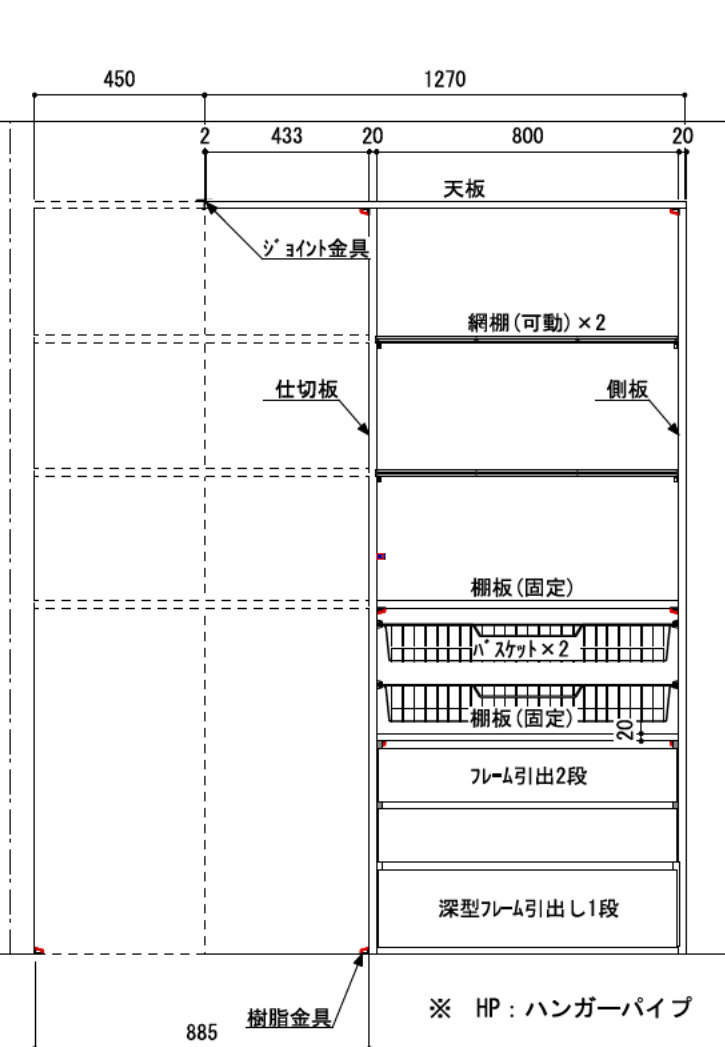
③立面
