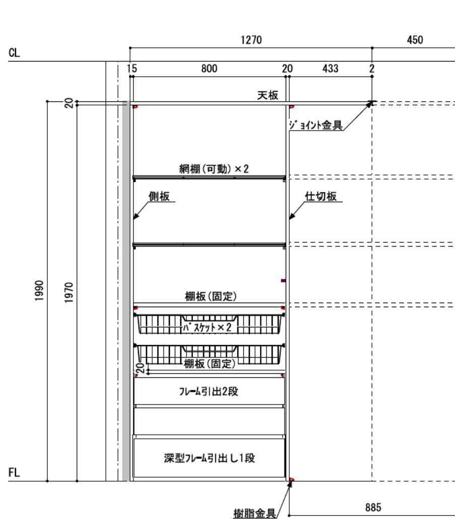
①立面
