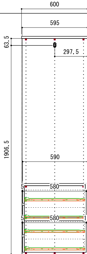
B-B' 断面
