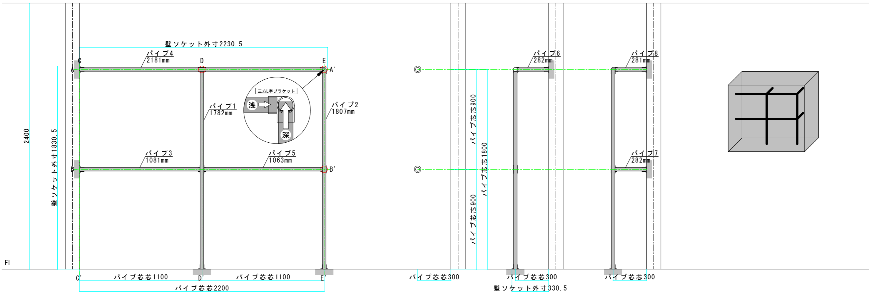
C-C' 断面
