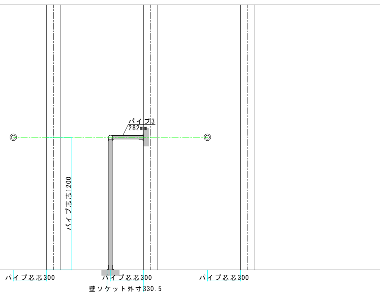
B-B' 断面
