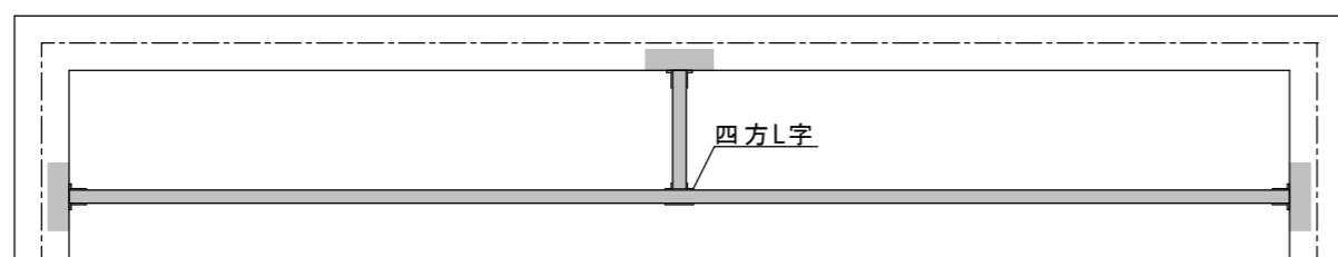
A-A' 平面
