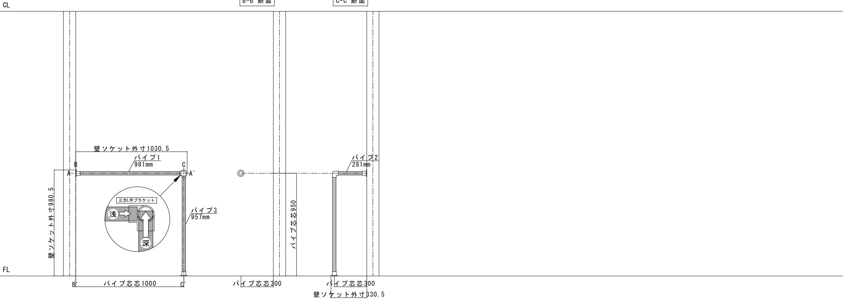
B-B' 断面
