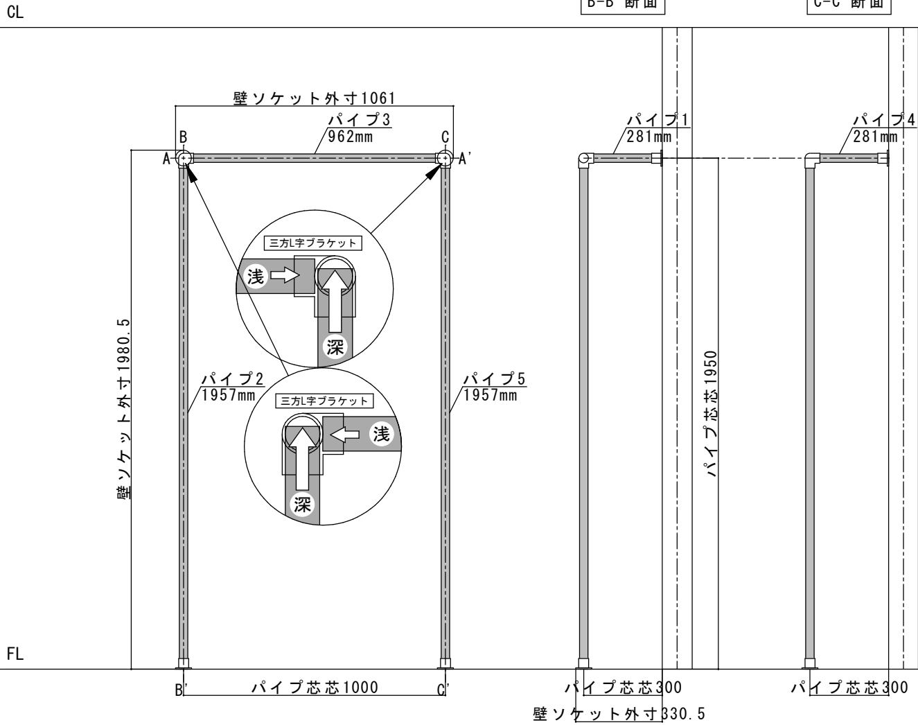
B-B' 断面
