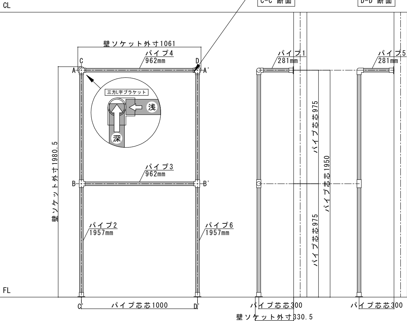
C-C' 断面
