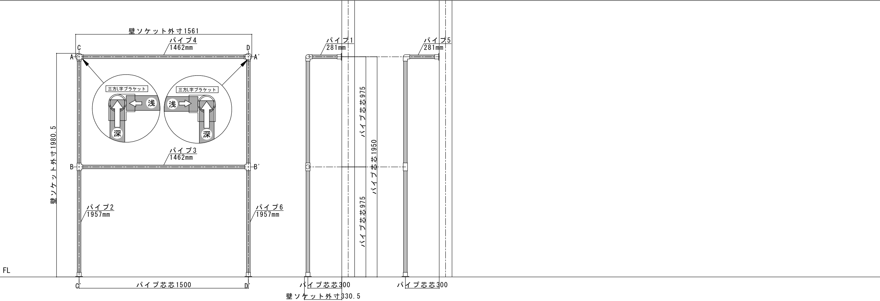
C-C' 断面
