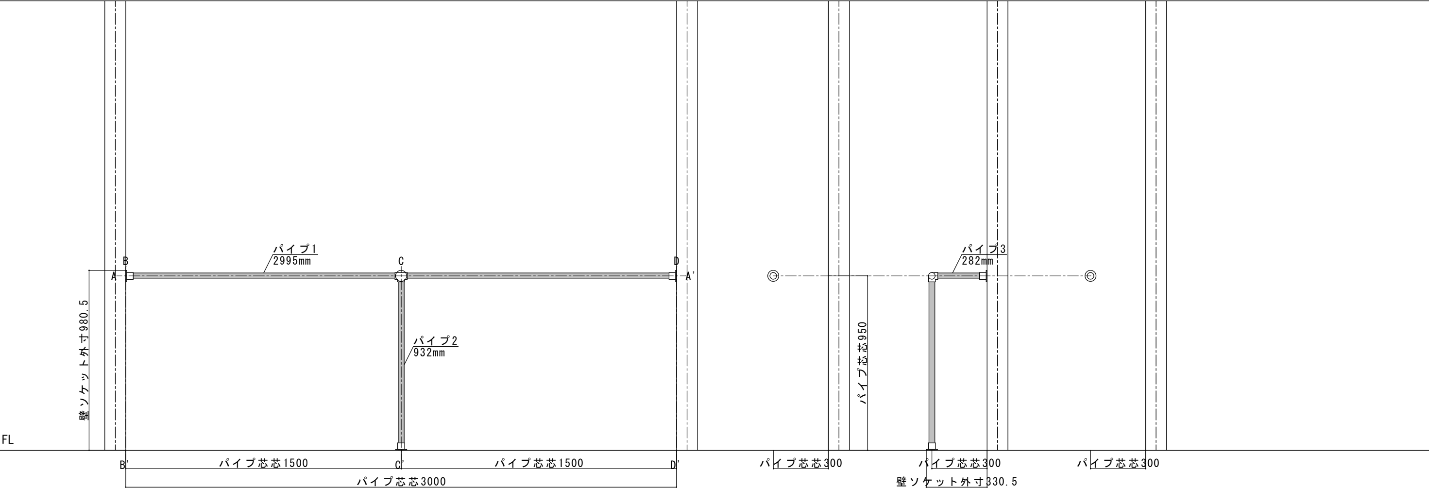
B-B' 断面
