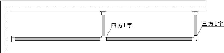
A-A' 平面
