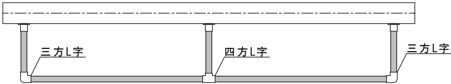
A-A' 平面
