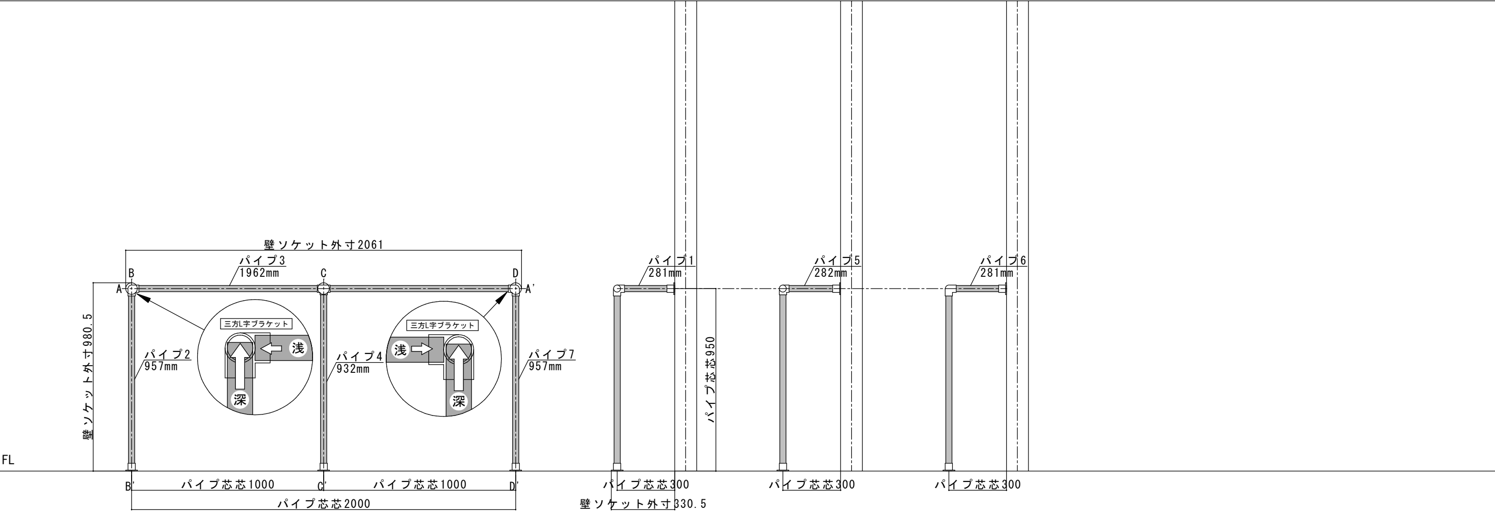
B-B' 断面
