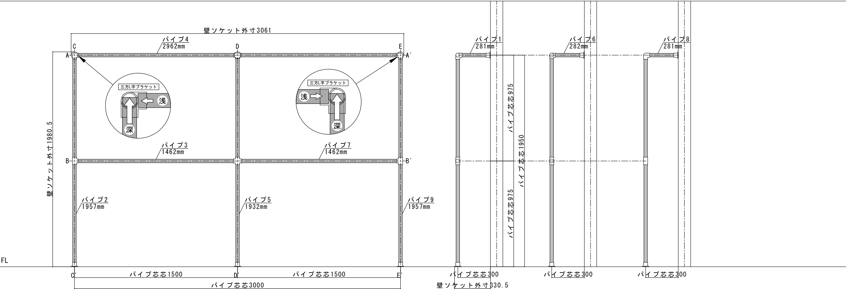
C-C' 断面
