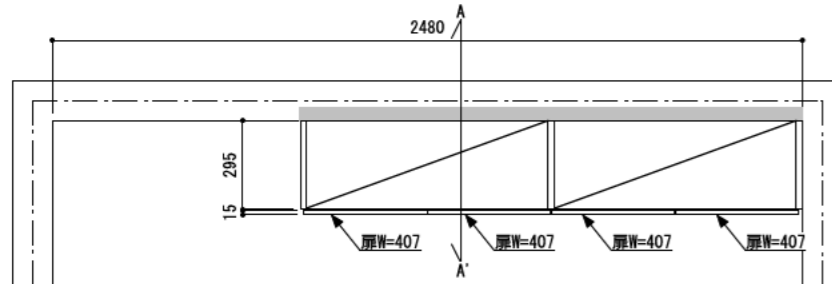
平面図（上部）
