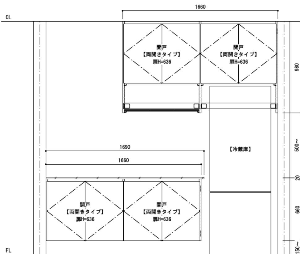
正面図（外観）
