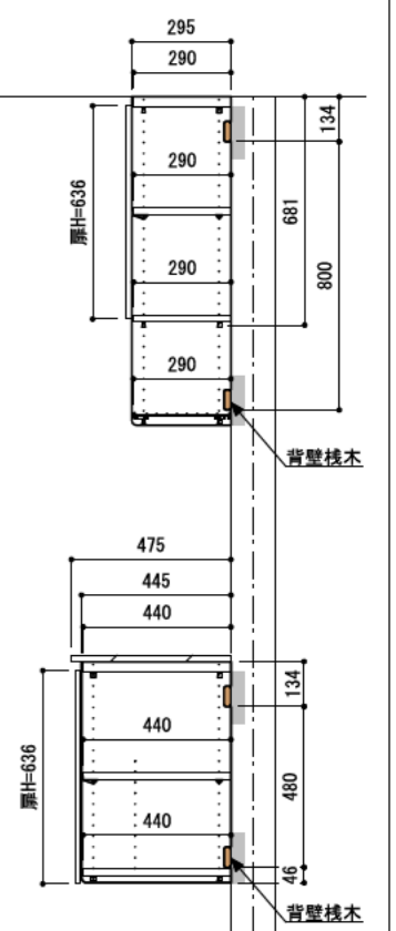
A-A' 断面
