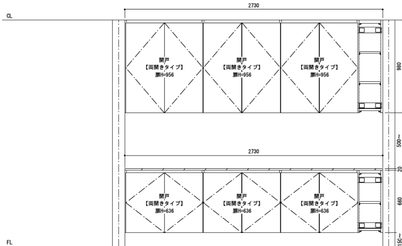
正面図（外観）
