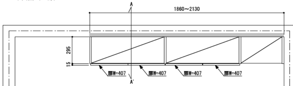
平面図（上部）
